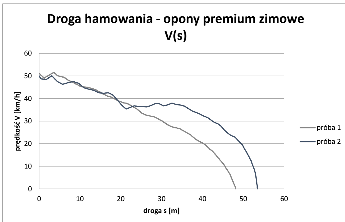
Wyk. 1. Przebieg procesu hamowania, opony premium zimowej
